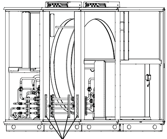
Jaetut peitelevyt putkien läpivientiä varten.
