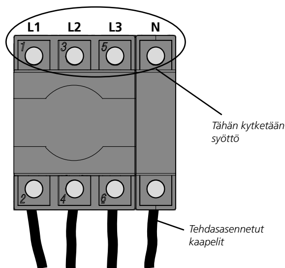
Turvakytkimen liitinrima.
