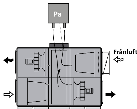
Princip för funktionen Air Quality Control (AQC).
