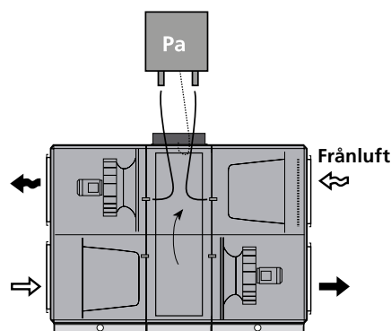
Princip för avfrostningsfunktion med separat tryckgivare.
