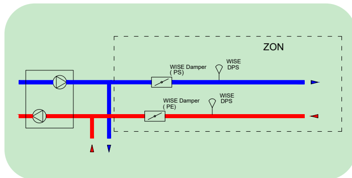
Principskiss, Konstanttrycksreglering
