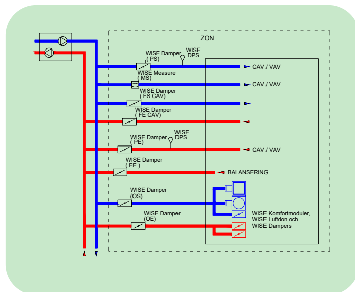
Principskiss, Flödesbalansering
