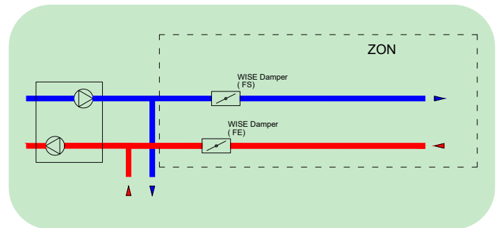
Principskiss, Konstantflödesreglering
